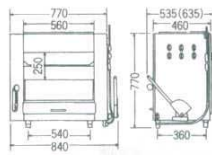
( ) 内寸法はレバーを下げた状態の寸法
