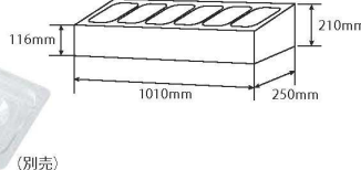
⑧18-8 テーブルトップサラダバー (6ホール) ステンレスGNインサート 100mmセット ㊦
