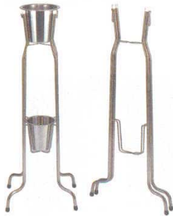
① フラワースタンド 折りたたみ式 18-8 8040400 S-1 480×340×H1,240 花入れ：上 φ220×φ170×H205 下 φ174×φ135×H165
