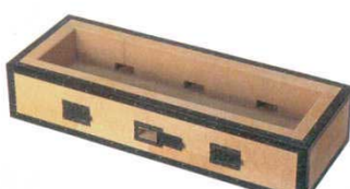
22 バーベキューコンロ BQ22号 炭用 6559700 外寸: 930×350×H210 内寸: 800×215×H115 重量: 25kg 付属品: 焼アミ
