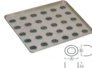
⑧天板 リージェント型 シリコン加工 (30ヶ取) 6739900 545×395×H49 単品寸法: A47 B33 H29
