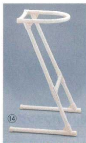
洗面器スタンド イレクター EBM 外寸 商品コード ⑭シングルタイプ 450×440×H750 8380700 ⑮ダブルタイプ 775×335×H750 8380800 ※32cmの洗面器が使用できます。 ※ダブルタイプはキャスター付です。 ※錆に強く、丈夫で軽い。 ※鋼鉄パイプに樹脂コーティング。
