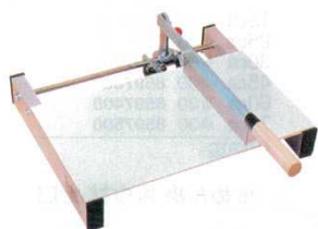
⑪ 麺切台
