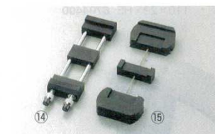
⑭ 砥石台 バイス式 280×70 0609900 ※最小18cm～最大21.3cmまでの砥石が入ります。
