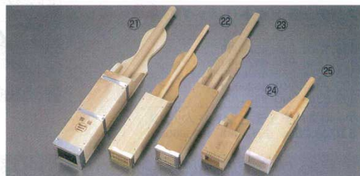
㉑ 天突 1812 業務用(特上) 木製 内寸：46×39×全長475 3542100 材質：刃/ステンレス板
