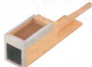
545×140×H170 0231300 上・(挿入口) 内寸法：190×100 下・(出口) 内寸法：102×102 出来上がり寸法 (個数)： 12×12×H12 (64個) 12mm角の寒天が64個出来上がります。
