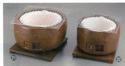
⑪ 三河コンロ大型 (茶) ⑫ 三河コンロ (茶) 5869000 5869100 外寸：φ270×H165 外寸：φ220×H165 付属品：焼杉敷板、焼アミ 付属品：焼杉敷板、焼アミ
