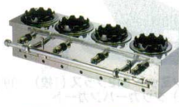
⑪釜めしガス炊飯器 一列 4個用
