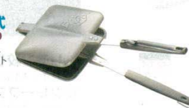
⑬ サンドイッチトースター XBW-02 ダブル 2723700 外寸：142×350×H37 焼き上がり寸法：65×115 ※内面フッ素樹脂加工
