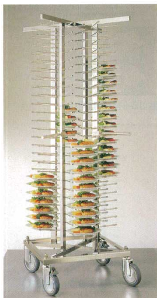
③ディッシュスタック 100 ユニバーサル EBM 4589100 皿にのせるバーが簡単に取り付け、取りはずしができる為、盛り付けにボリュームがあっても対応します。また単一の料理だけでなくその状況に合わせて必要箇所だけ取りはずせば良いので省スペースを考えてディッシュスタックの中の省スペース化モデルです。 ※φ18cm～33cmの皿が使用できます。 ※キャスターφ150 4輪自在 (内2ヶストップバー付)
