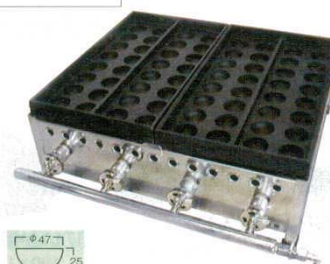
⑩ たこ焼機 ジャンボ 32穴 直 A 抗腐 ガス接続口：LPφ9.5・都市ガスφ13
