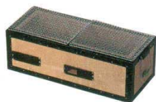
①バーベキューコンロ BQ8WF号 炭用 6559500 外寸：540×230×H200 内寸：460×150×H110 重量：10kg 付属品：焼きアミ
