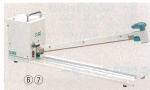
⑥卓上シュアーシーラー NL-450K 1126900 外寸：649×124×H238 重量：7.0kg 電源：単相100V 消費電力：650W シーリング時間：0.2～1.5秒 シール寸法：2.5mm巾×450
