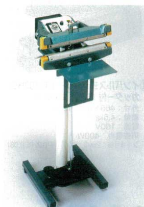
⑫シーラー インパルス CHB-300 スタンド式 8775200 外寸：370×330×H900 最大フィルム幅：300 電源：単相100V / 400W 重量：27kg ●インパルス方式
