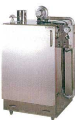
⑤ スモーク薫製機 SU-50F ¥974,000 f 外形寸法:W970×D730×H1,550mm 内形寸法:W700×D630×H780mm 重量:168kg 電源:三相200V 3.16kW 送風機 0.06kW ヒーター 3kW 機器0.1kW 装置:サーモ、温度計 付属品:棚網2枚、丸棒4本 ※重気ファン式、攪拌対流
