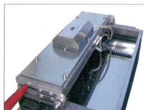
※たい焼き板背面にヒーター密着タイプ
