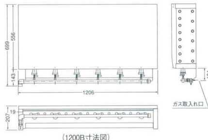
(1200B寸法図)
