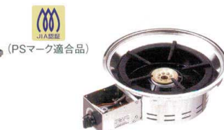
2 器具ユニット(鍋用) CTK-22S c LP ¥45,000 13A ¥45,000 燃焼器寸法:W460×D380×H152mm ガス消費量:LPG 3.21kW (0.23kg/h) 13A 3.14kW (2700kcal/h) 点火方式:圧電点火方式 天板開口寸法:φ348mm ガス接続口:LP・13A:9.5mmホース用ホースエンド 使用可能最大鍋径:26cm
