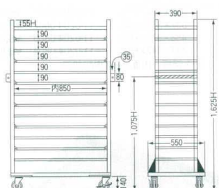
⑩ 食パン6取兼用 26枚差ラック オールステンレス [DTRK-01]
