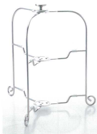
ワンタッチプレートスタンド ¥10,000 (税抜価格) 適合プレート: 19cm~24cm 製品寸法 (折りたたみ時): 180×296×50mm (使用時): 310×296mm 材質: ステンレス製 品番: SK455-1
