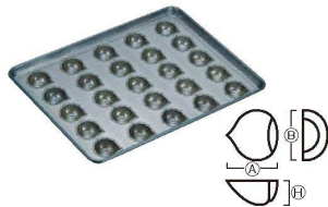
⑦シリコン加工 マロンケーキ型 天板 (25ヶ取) 6739600 ¥22,500 外寸:545×395×H53 単品寸法:①59 ②59 ③30
