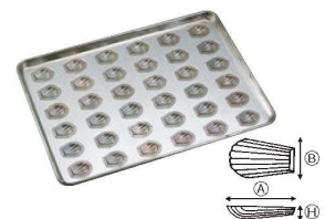
③シリコン加工 貝形マドレーヌ型 天板 小 (36ヶ取) 5396700 ¥24,600 外寸:545×395×H34 単品寸法:①43 ②33 ③12
