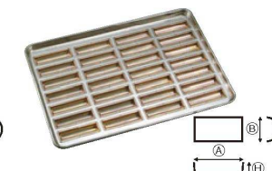
⑯シリコン加工 ラフト型 天板 M (28ヶ取) 5396100 ¥24,600 外寸:545×395×H38 単品寸法:①110 ②26 ③16
