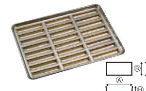
⑮シリコン加工 ラフト型 天板 (24ヶ取) 5396000 ¥24,600 外寸:545×395×H38 単品寸法:①150 ②26 ③18
