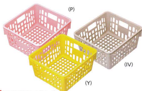
新 PSK-300N 食器かご 390×360×200 ¥7,400 内寸(底面) / 333×301×186 重量 / 945g
