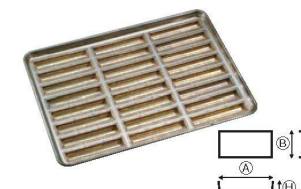
⑮シリコン加工 ラフト型 天板 (24ヶ取) 5396000 ¥25,000 外寸:545×395×H38 単品寸法: A150 B26 H18
