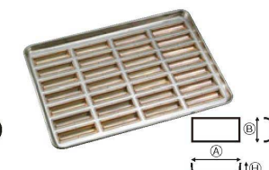
⑯シリコン加工 ラフト型 天板 M (28ヶ取) 5396100 ¥25,000 外寸:545×395×H38 単品寸法: A110 B26 H16
