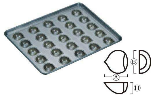
⑦シリコン加工 マロンケーキ型 天板 (25ヶ取) 6739600 ¥22,500 外寸:545×395×H53 単品寸法: A59 B59 H30
