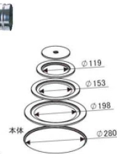
② クッキングストーブ RS-41 0935600 ¥18,000 430×350×H940 (H450) 重量: 6.9kg 材質: 鉄鋼板 使用燃料: 薪
