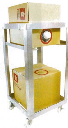
5 アルミ製 エーステナー台車W型 2缶用 〈HDI-80〉目 7-1456-0501 ¥48,000 396×396×H785 キャスター:ナイロン製φ75×4自在 2輪スッパ付 ●エーステナー 295×295×H285(20ℓ)×2用
