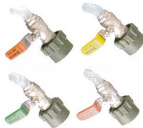
8 一斗缶用バルブ MWC-40BS 〈KBL-41〉目 ¥8,700 7-1456-0801 赤 7-1456-0802 緑 7-1456-0803 黄 7-1456-0804 オレンジ ●スカート(盛りあがり口)外寸φ40mm専用。 ●ワンタッチ脱着で液こぼれがなくスムーズに注ぐことができます。 ●中身がわかりにくい液体をレバーの色で区分けできます。
