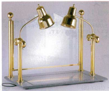
2 カービング ディスプレイ ヒートランプウォーマー 2灯タイプ 〈NLV-15〉 7-1538-0201 ¥492,000 910×510×H760 電源:単相100V 消費電力:500W (250W×2) ※ランプの角度が自由に調節できます。
