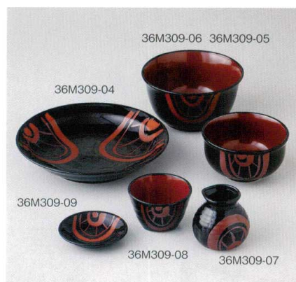
御所車
