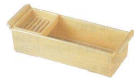
11-351-8K シャンプー箱 ¥ 3,150 W327・D120・H90 目皿付き ABS ウレタン塗装
