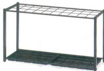
11-561-12 組立 ¥22,400 (W920・D300・H500) 本体：スチールに粉体塗装(ブラック) 傘枠：スチールに粉体塗装(ブラック) 受皿：樹脂成型品(ブラック)、大2枚
