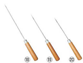
先丸千枝通し 全長 商品コード 価格 ⑱大 TS-160 290 6794400 ¥560 ⑲中 TS-161 240 6794500 ¥530 ⑳小 TS-162 215 6794600 ¥500 ●鉄板などの表面をキズつけにくい先丸加工
