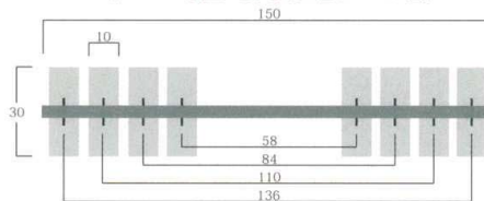
《W150cm衝立 脚可動位置イメージ図》
