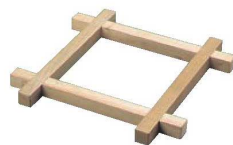
⑨木製 だしこし用 井ゲタ ページコード 商品コード 価格 2-0584-0901 5720900 ¥11,400 外寸:450×450×H35 内寸:270×270
