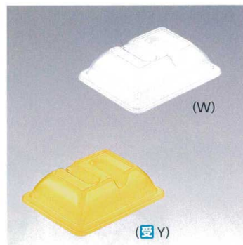
C-1612 164 × 128 × 45 ¥470 (適応食器 KS-865 / MS-870 / MS-873 / MS-875)
