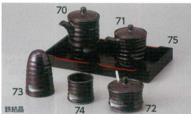
鉄結晶
