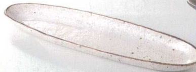
熔岩流
