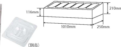
⑧18-8 テーブルトップサラダバー (6ホール) ステンレスGNインサート 100mmセット
