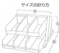
⑭ BK オーガナイザー 3段2列 O-3-2-B ブラウン [FOGN-15] U 13-0436-1401 ¥17,500 サイズ：(A)315×(B)565×(C)355
