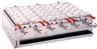
② 蜜元式 焼饅頭機 KMG-3A(3連)
