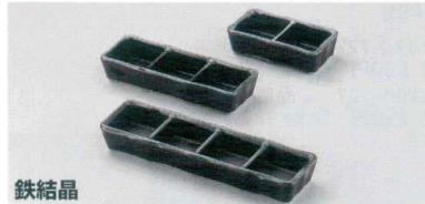
鉄結晶
