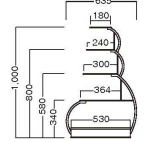
3 UK18-8 5段 ウェディング ケーキスタンド A 0206 0015 〈NKC-60〉 9-1769-0301 ¥450,000 635×φ530×H1,000
