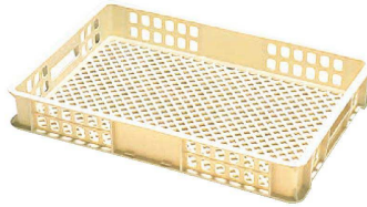
⑤ セキスイ コンテナ BT-22 〈AKV-E2〉 洗 9-0188-0501 ¥4,280 内容量:22ℓ 外寸:645×428×H95 内寸:610×400×H89
