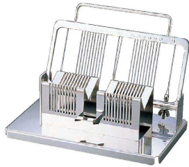
1 2連横型エッグカッター 〈BTM-37〉 9-0571-0101 ¥120,000 170×178×H90 質量:1.38kg 材質:ステンレス ●替ワイヤー1セット付(2本)。
