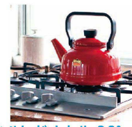
⑭ ソリッド ケトル 2.3ℓ SD-2.3K <ASL-72> ¥5,000 9-0064-1401 R 赤 9-0064-1402 SB 青 外径 口径 高さ 底径 185 95 160 150
