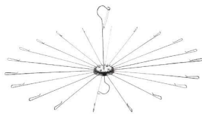
⑤ステンレス パラレルハンガー 20本 SHP-20 ページコード 商品コード 価格 4-2374-0501 1246800 ¥5,000 外寸:φ810×H390 重量:750g 収納時:φ92×H490 バーの長さ:360 ●落下防止の先端クリップ形状 ●折りたたみ式 ●フックストッパー付
