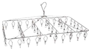
⑨ステンレス 角型ピンチハンガー 48ピンチ SHS-48F ページコード 商品コード 価格 4-2374-0901 1073650 ¥5,000 外寸:700×390×H295 重量:1,050g 収納時:360×390×H50 ●向きが変えられ干しやすい360度回転式フック ●折りたたみ式なので、収納時はコンパクト ●折りたたんでもピンチとピンチが密に合い両吊り仕様
