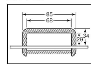
フック寸法
