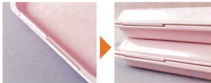
■ トレー重ね時の短手凹凸組み合わせ
