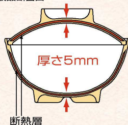
■製品断面図
