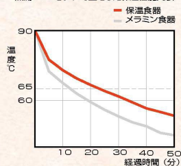
■保温性能テスト 室温:23℃ 熱湯90℃をいれて蓋をした保温性能実験
