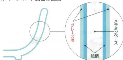
ダブルコーティング食器断面図
